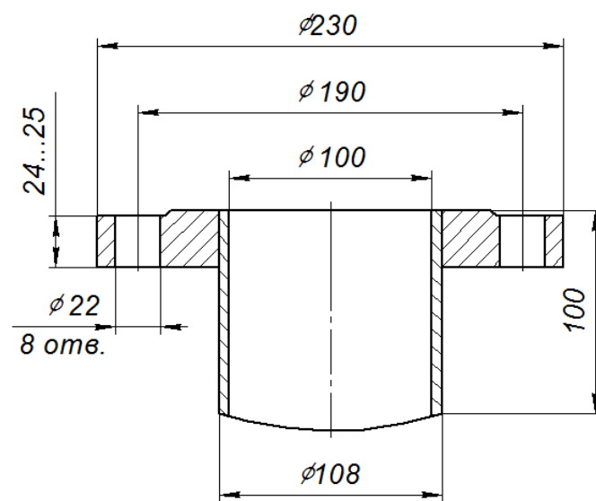
Размеры приварного патрубка на давление 2,5 МПа
