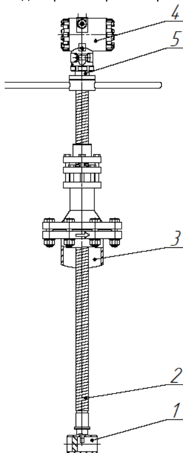
Рисунок 1.1 – Устройство погружного расходомера
