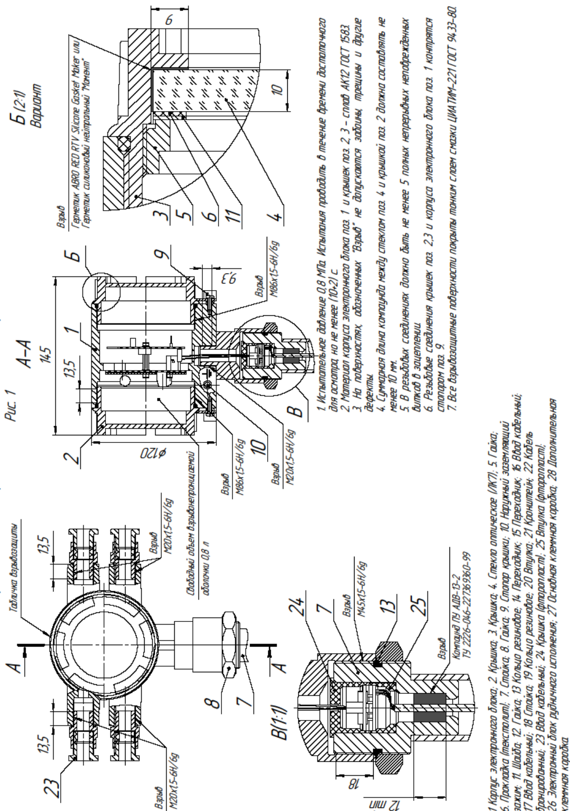
Электронный блок с четырьмя клапальными валами интегрального исполнения
