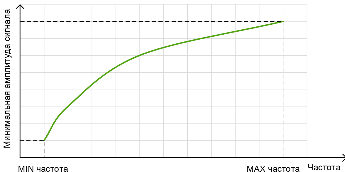
Рисунок 9.12. Зависимость минимальной амплитуда полезного сигнала от частоты
