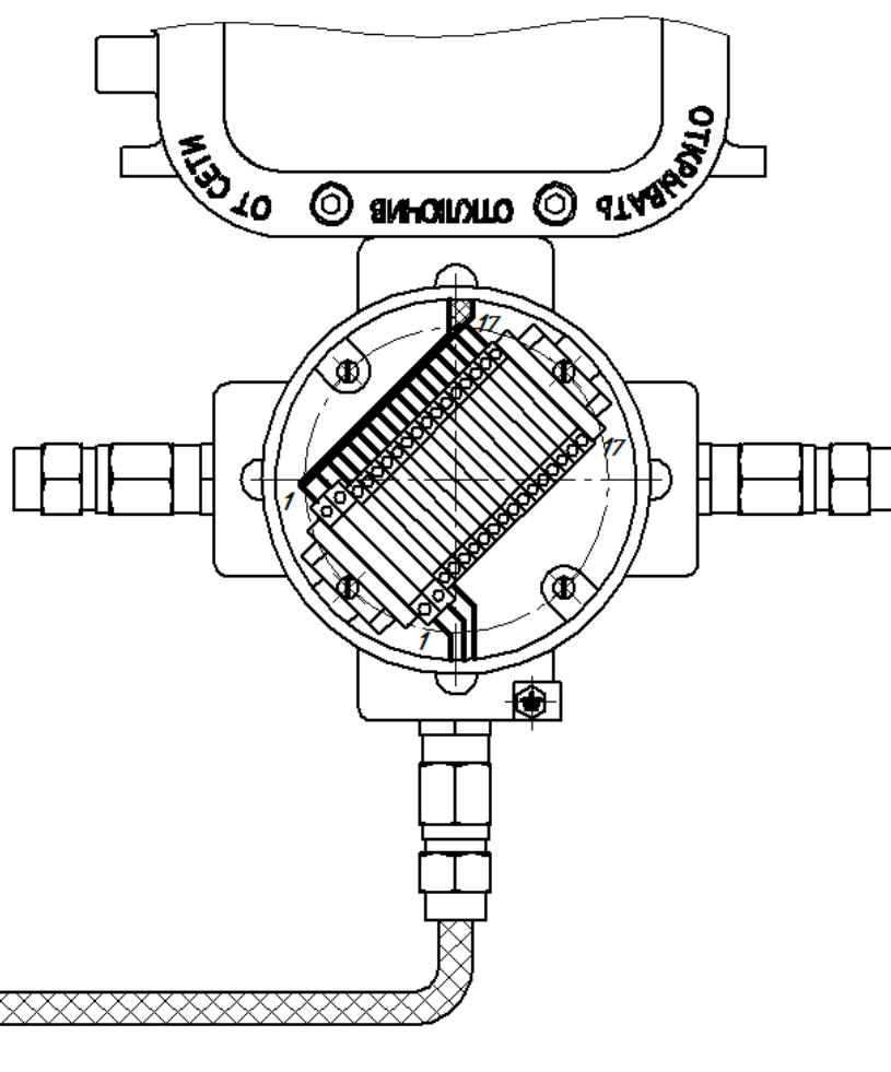
Рисунок В.3 - Расположение зажимов клеммной колодки для взрывозащищенного исполнения РВ с рудничной взрывозащитой
