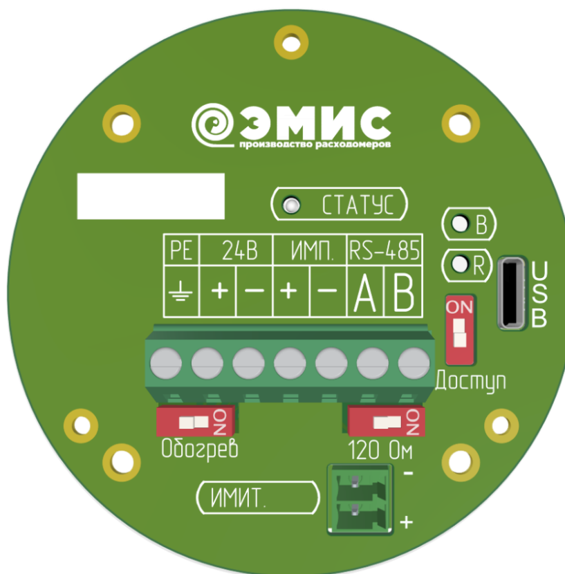
Рисунок 7.1. Плата клемм
