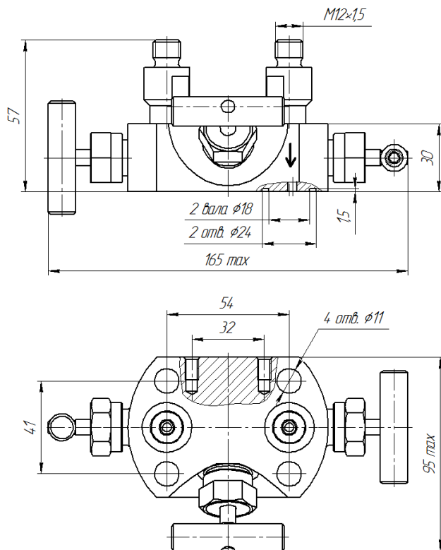
Рисунок А.9 – Габаритно-присоединительные размеры и гидравлическая схема 3-вентильных блоков исполнения БКНЗ-11-12С
