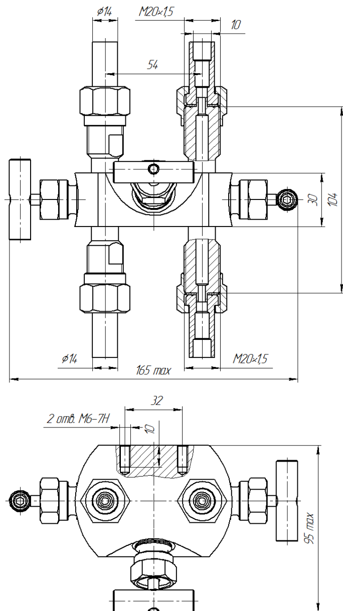
Рисунок А.11 – Габаритно-присоединительные размеры и гидравлическая схема 3-вентильных блоков исполнения БКНЗ-11-20П2
