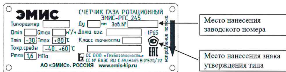
Рисунок 2 – Места расположения знака утверждения типа и заводского номера счетчика на маркировочной табличке
