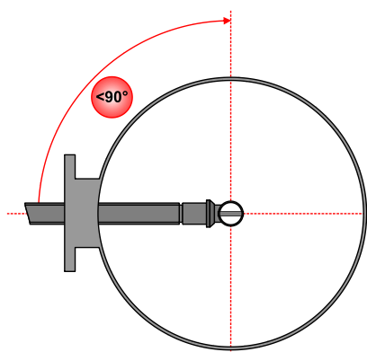
Рисунок 2.2 – Угол установки расходомера
