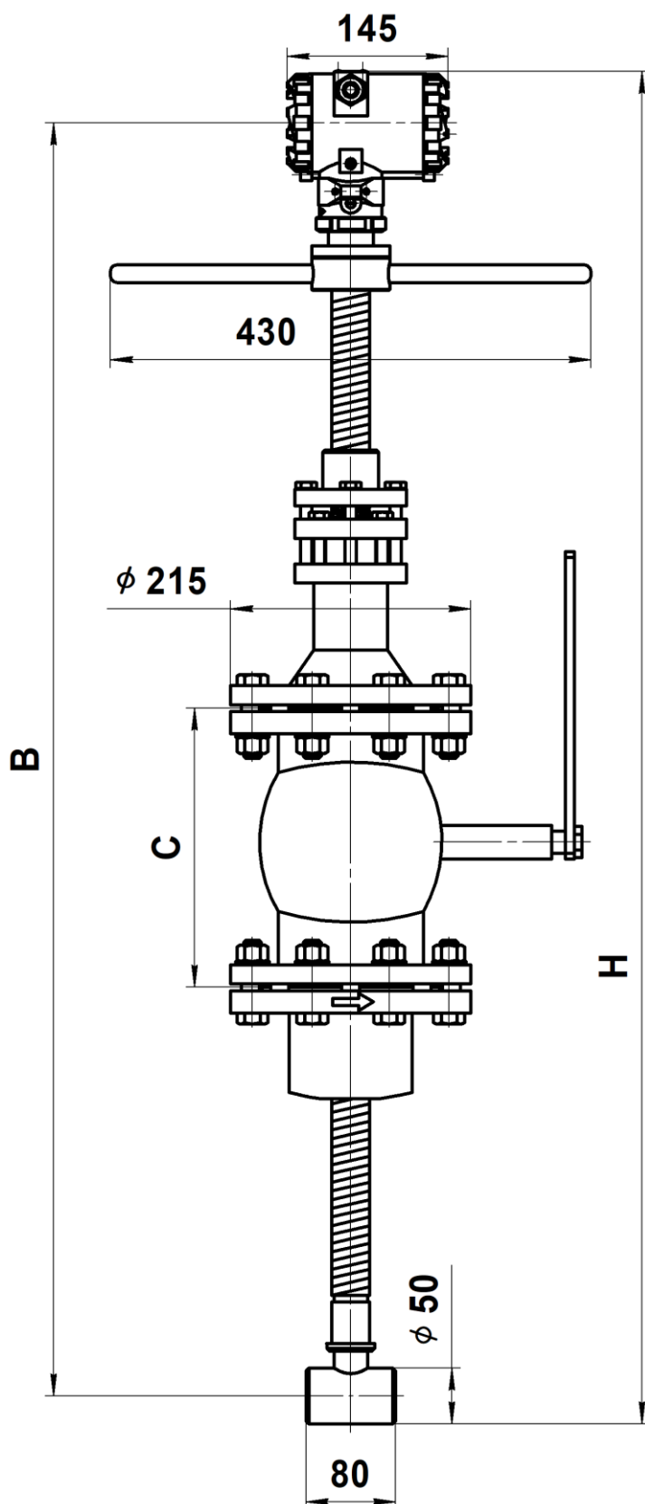
Рисунок Б.1 – Размеры погружного расходомера на давление 1,6 МПа исполнения «-»
