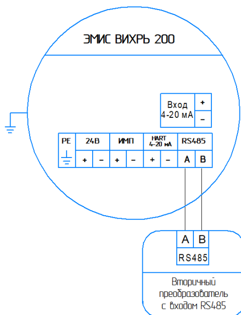
Рисунок 8.10. Схема подключения электронного блока к вторичному оборудованию по интерфейсу RS485
