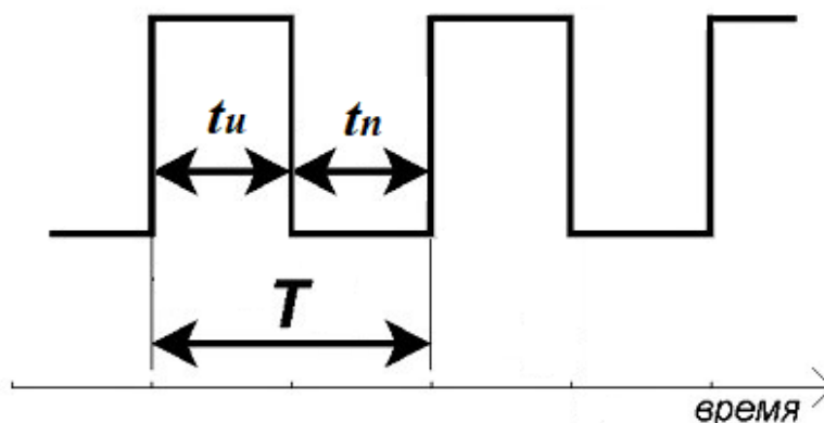
Рисунок 7.3 – Сигнал на частотно-импульсном выходе при t_u = t_n
