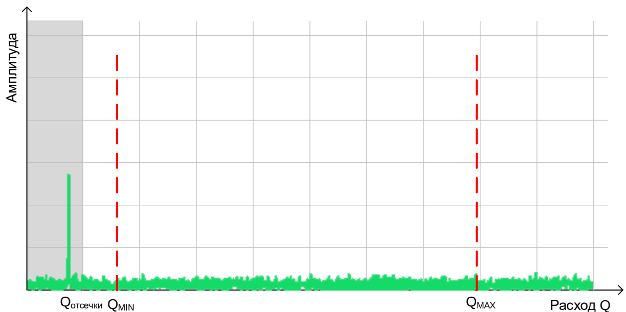
Рисунок 9.17. Отсечка по минимальному расходу
