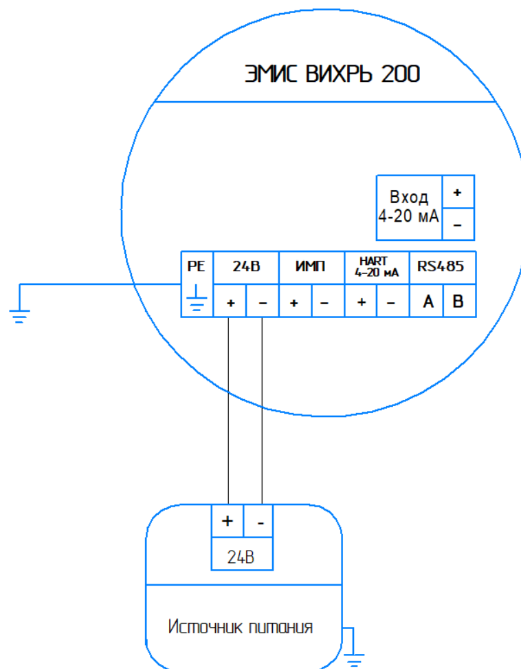
Рисунок 8.4. Схема подключения питания
