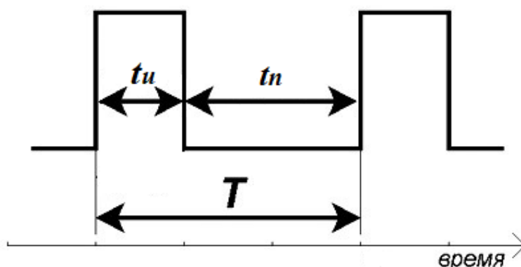
Рисунок 7.2 – Сигнал на частотно-импульсном выходе при t_u < t_n
