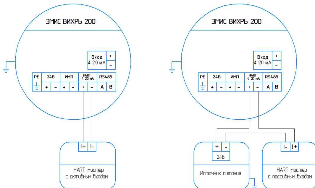
Рисунок 8.8. Схема подключения электронного блока к HART-мастеру с активным (слева) и пассивным (справа) входом цифрового протокола HART
