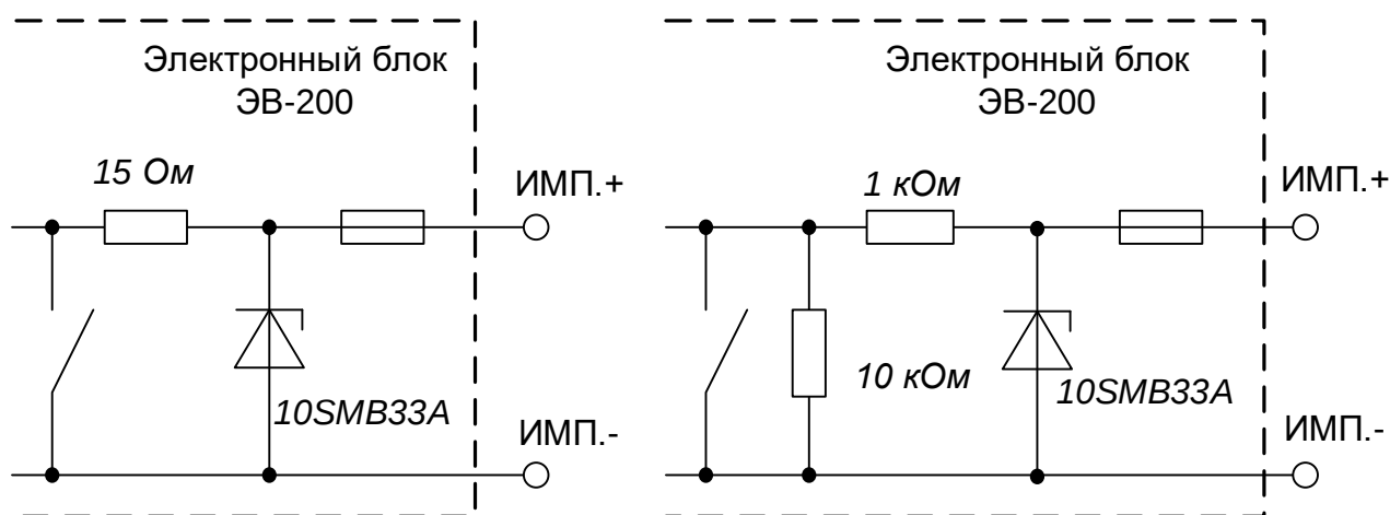
Рисунок 7.1. Принципиальные схемы частотно-импульсного стандартного выхода (слева) и NAMUR NA01 (справа)
