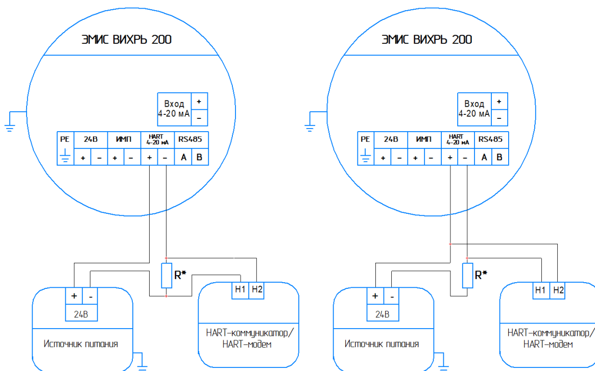
Рисунок 8.9. Схема подключения HART-коммуникатора или HART-модема к электронному блоку для работы по протоколу HART
