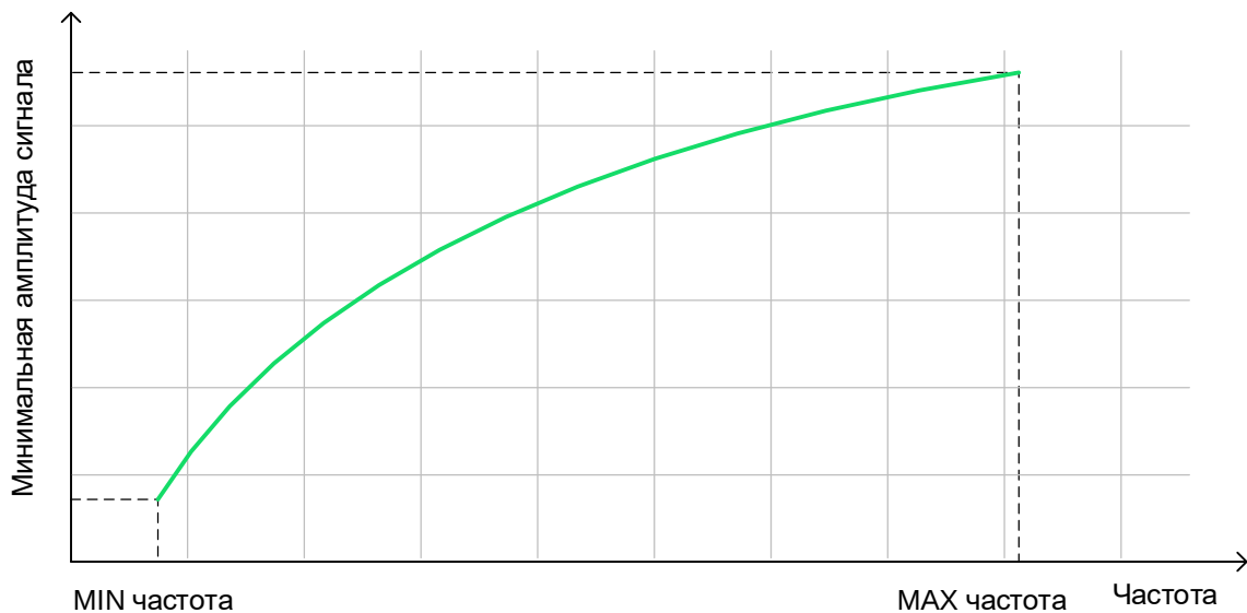
Рисунок 9.12. Зависимость минимальной амплитуды полезного сигнала от частоты
