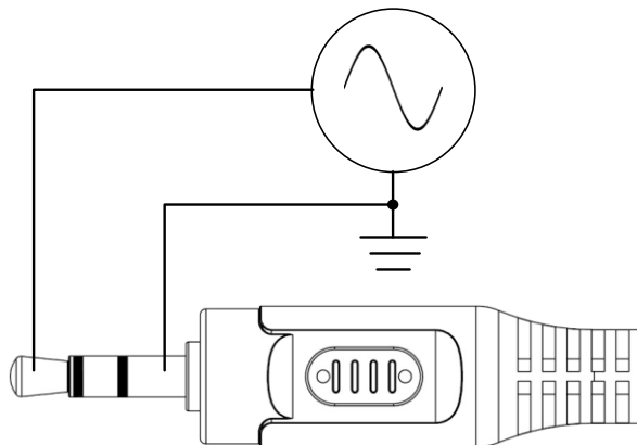
Рисунок 11.1. Схема подключения внешнего генератора к аудио штекеру
