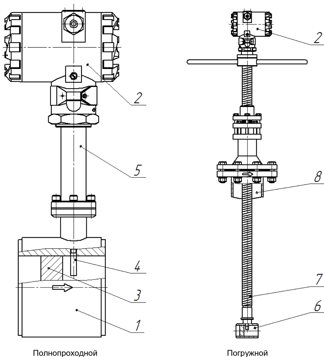
Рисунок 3.1. Устройство расходомеров расхода
