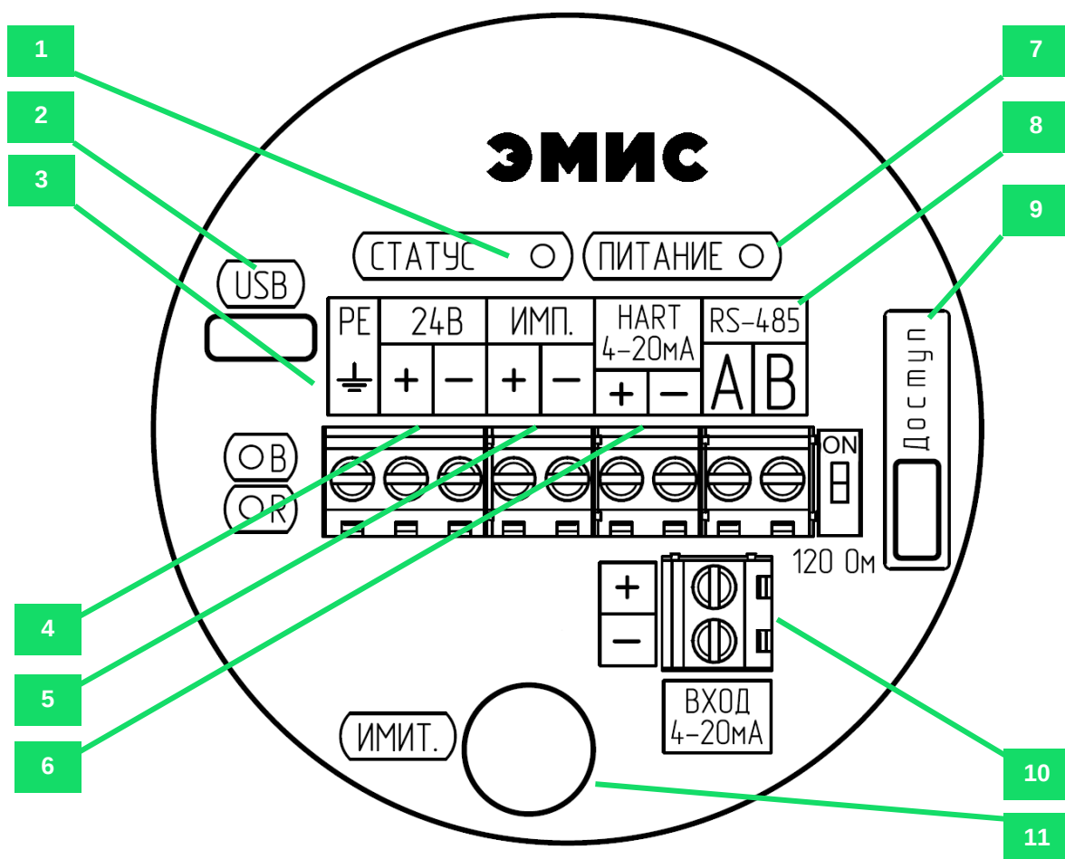
Рисунок 8.1. Плата интерфейсов электронного блока
