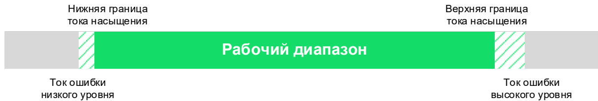
Рисунок 7.5 Диапазоны токов датчика давления
