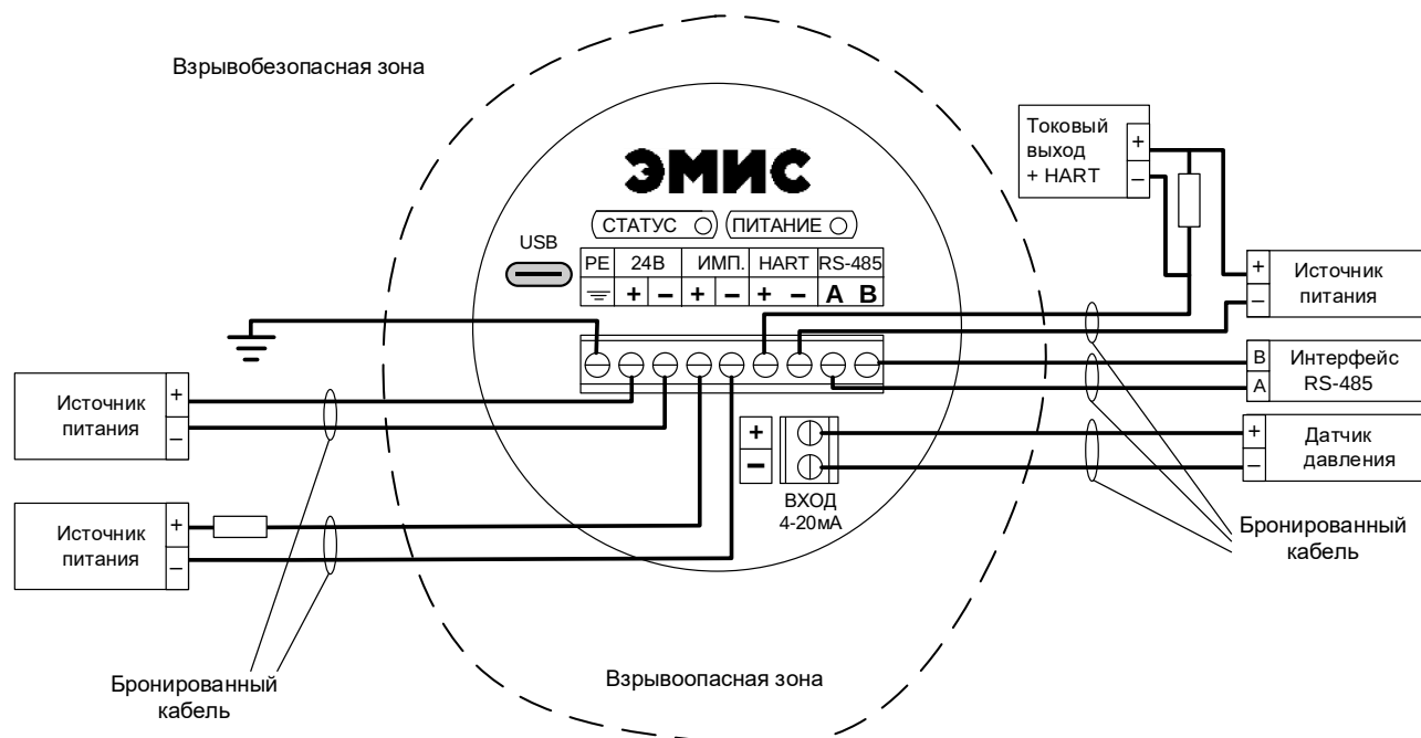
Рисунок 8.13. Пример схемы подключения расходомеров взрывозащищённых исполнений Вн и ВнIII с видами взрывозащиты «d» и «t» соответственно
