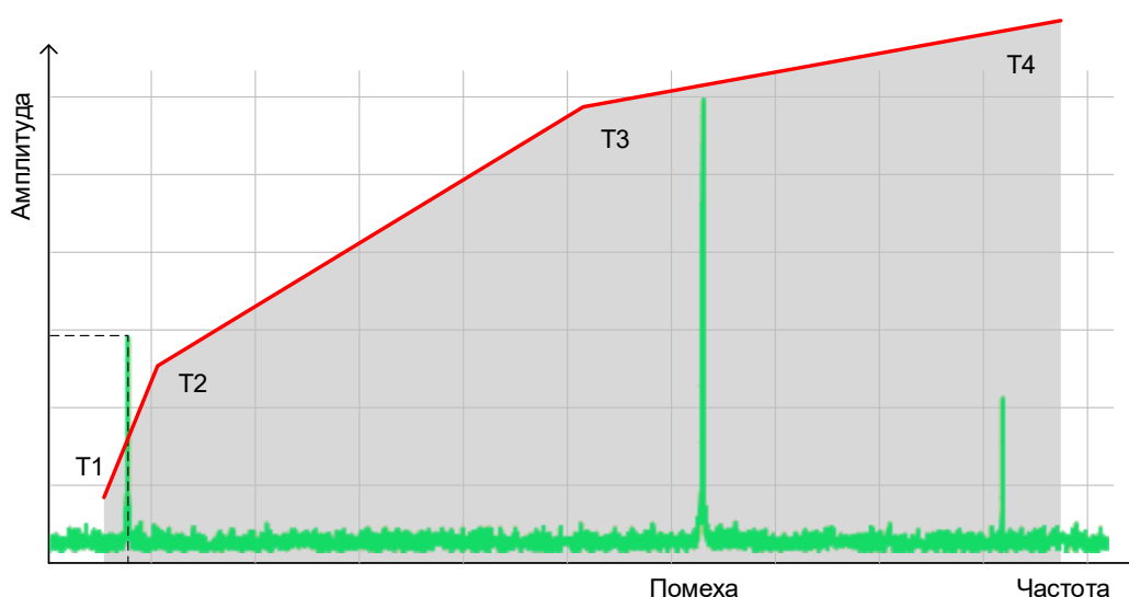
Рисунок 9.15. Фильтрация сигнала адаптивным фильтром
