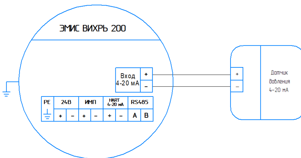
Рисунок 8.11. Схема подключения датчика давления к электронному блоку
