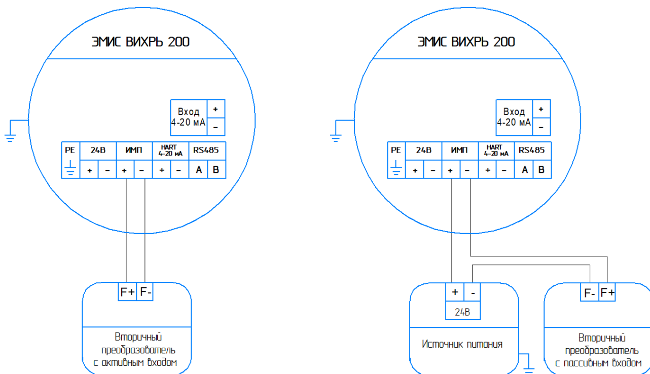
Рисунок 8.6. Схема подключения частотно-импульсного или дискретного выхода электронного блока к вторичному преобразователю с активным (слева) и пассивным (справа) частотным входом
