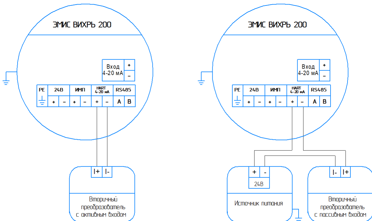
Рисунок 8.7. Схема подключения токового выхода 4-20 мА электронного блока к вторичному преобразователю с активным (слева) и пассивным (справа) токовым входом
