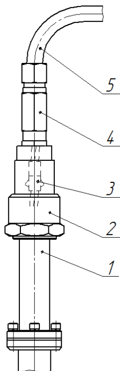
Рисунок 6.2. Разъёмное дистанционное исполнение
