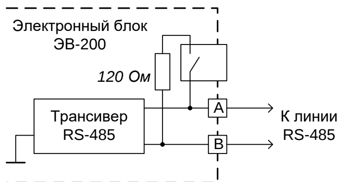
Рисунок 7.4. Схема подключения электронного блока по интерфейсу RS-485
