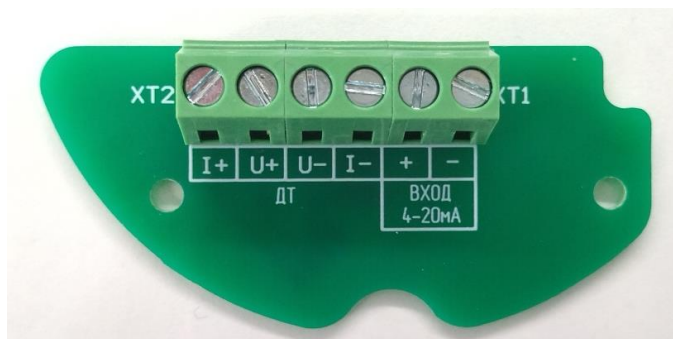
Рисунок 8.2 – Плата коммутации для подключения датчика давления и датчика температуры
