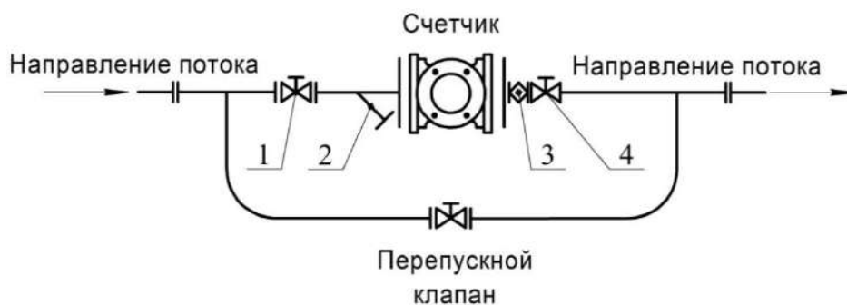
Рисунок 2.5 – Горизонтальная установка счетчика
