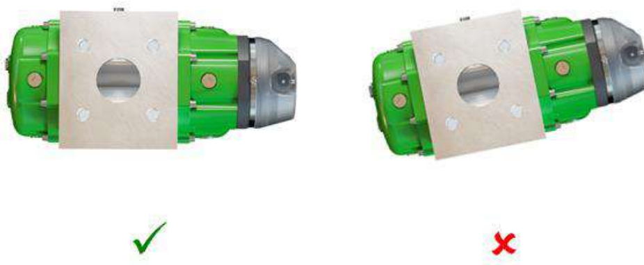
Рисунок 2.2 – Положение счетчика при монтаже на горизонтальном участке трубопровода
