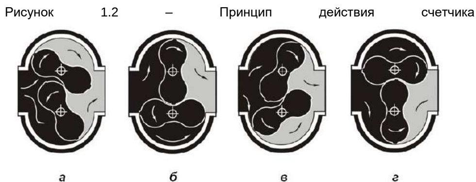
Рисунок 1.2 – Принцип действия счетчика
