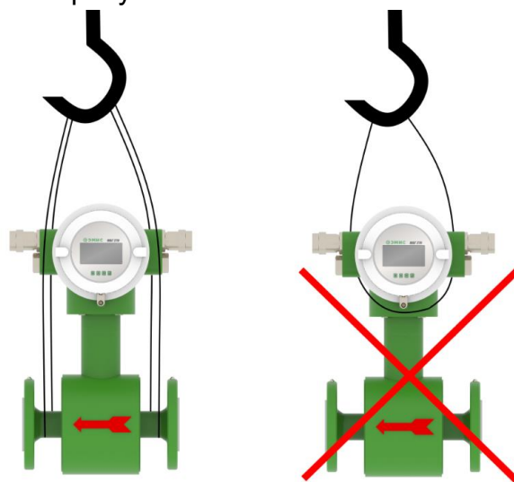
Рисунок 3.1 – Правила транспортирования счетчика-расходомера вне тары
