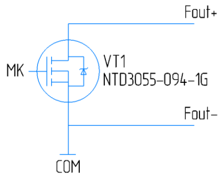
Рисунок 1.3 – Схема пассивного частотно-импульсного выхода расходомера ЭМИС-МАГ 270
