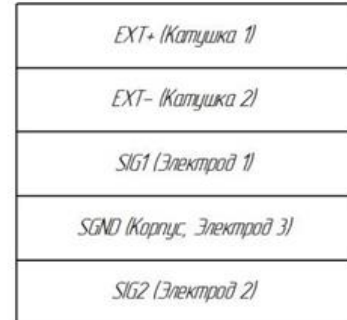
Схема клеммной колодки дистанционного исполнения
