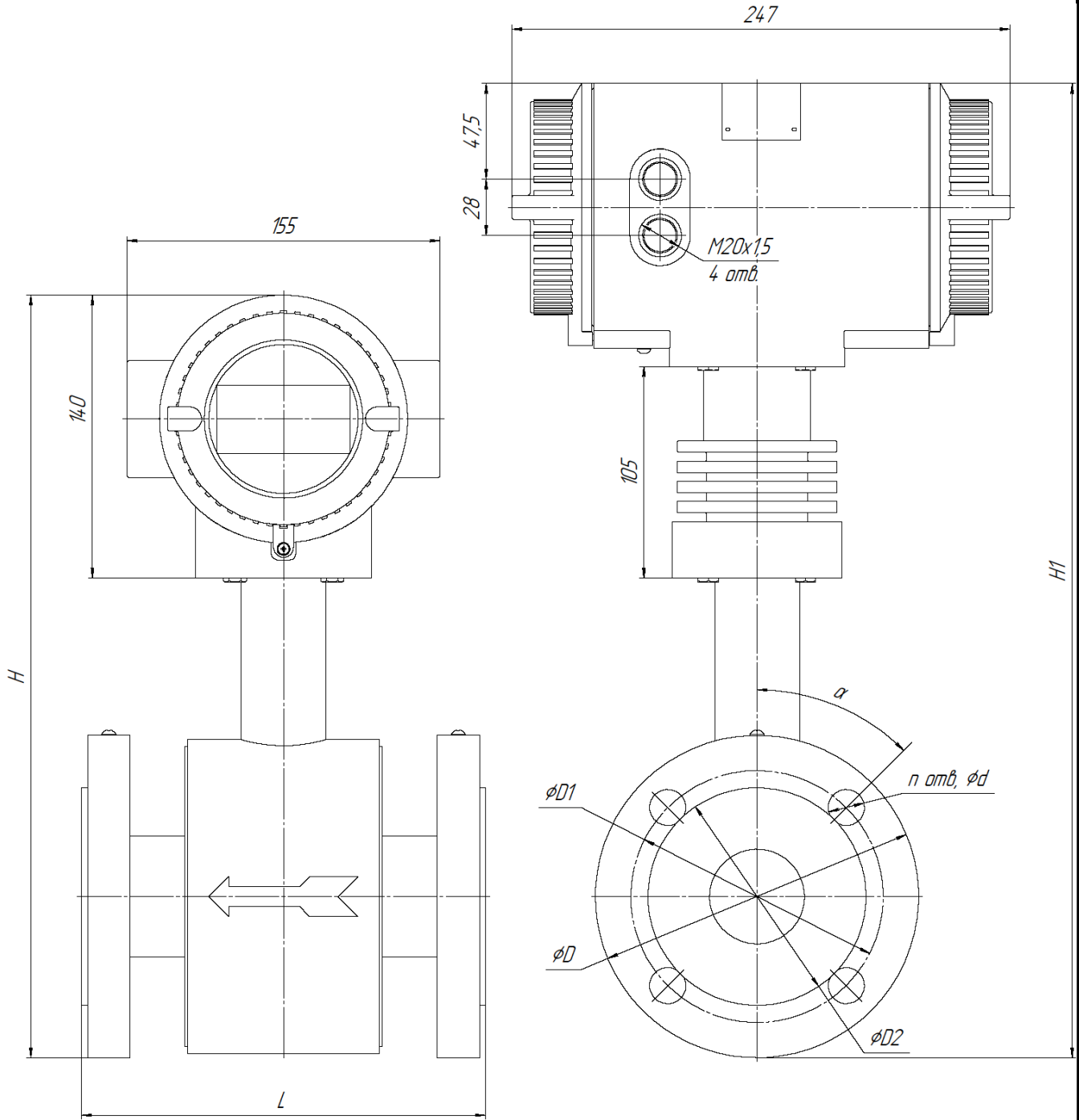
Рисунок А.1 – Габаритные и присоединительные размеры счетчика-расходомера интегрального исполнения (размер «Н») и интегрального высокотемпературного исполнения (размер «Н1») с фланцевым соединением с трубопроводом
