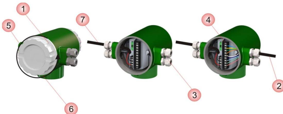
Рисунок 2.6 – Подключение электронного преобразователя
