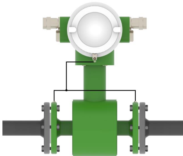
Рисунок 2.10 – Защита от переходных процессов при монтаже на токопроводящем трубопроводе
