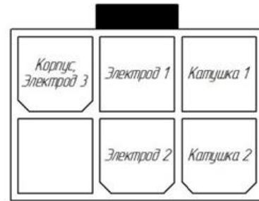
Схема разъёма интегрального исполнения
