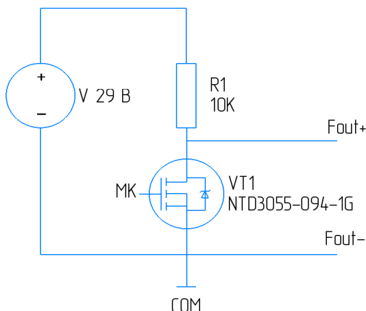
Рисунок 1.4 – Схема активного частотно-импульсного выхода расходомера ЭМИС-МАГ 270
