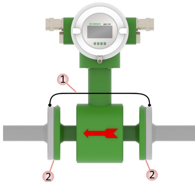
Рисунок 2.9 – Заземление счетчика-расходомера на трубопроводе с катодной защитой
