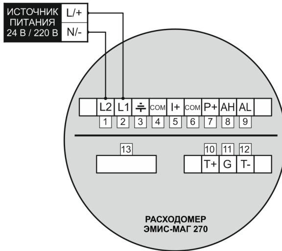
Рисунок В.2 – Схема подключения питания
