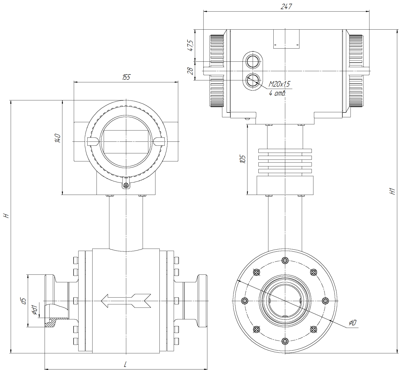
Рисунок А.3 – Габаритные и присоединительные размеры счетчика-расходомера интегрального исполнения (размер «Н») и интегрального высокотемпературного исполнения (размер «Н1») с муфтовым соединением с трубопроводом («молочная гайка» по DIN 11851)
