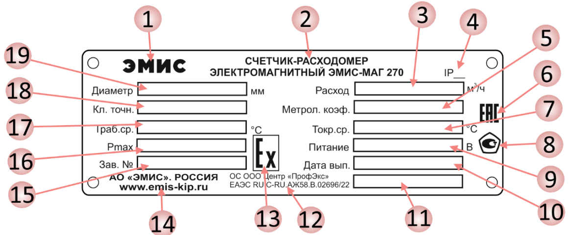
Рисунок 1.5 – Основная табличка счетчика-расходомера
