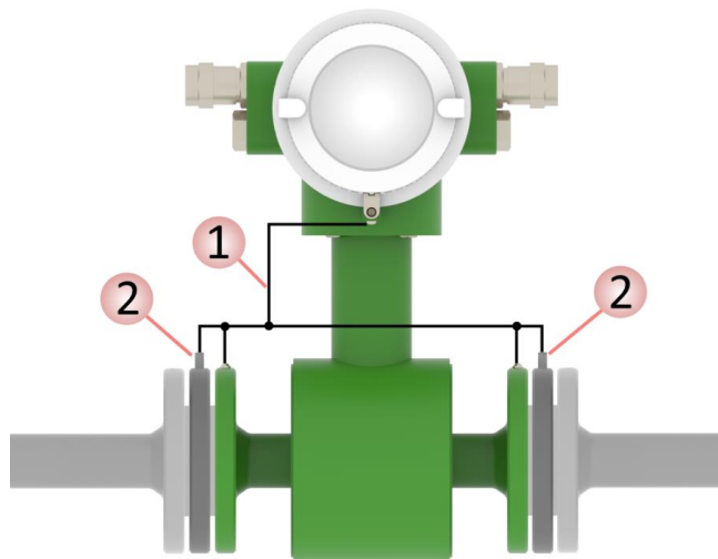
Рисунок 2.11 – Защита от переходных процессов при монтаже на трубопроводе из поливинилхлорида, фторопласта и других пластиковых материалов, на окрашенных трубопроводах или трубопроводах, имеющих внутреннее покрытие
