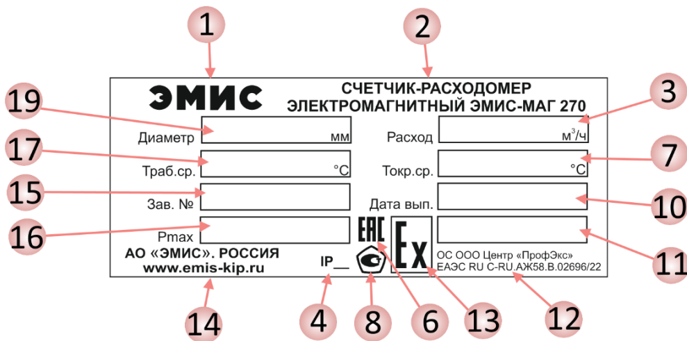
Рисунок 1.6 – Дополнительная табличка счетчика-расходомера
