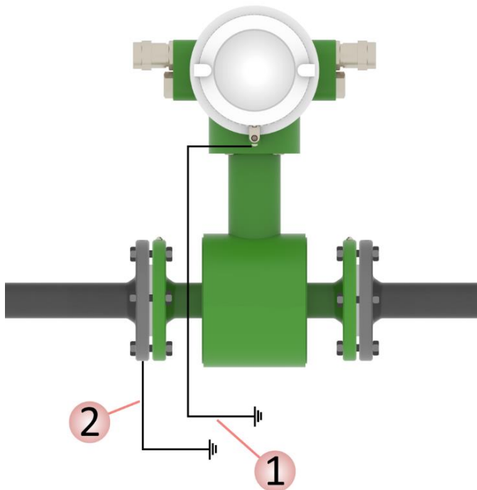
Рисунок 2.8 – Заземление счетчика-расходомера
